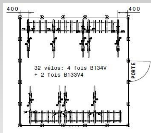
Implantation des vélos pour le modèle 5x5m réf. M107V5R0
